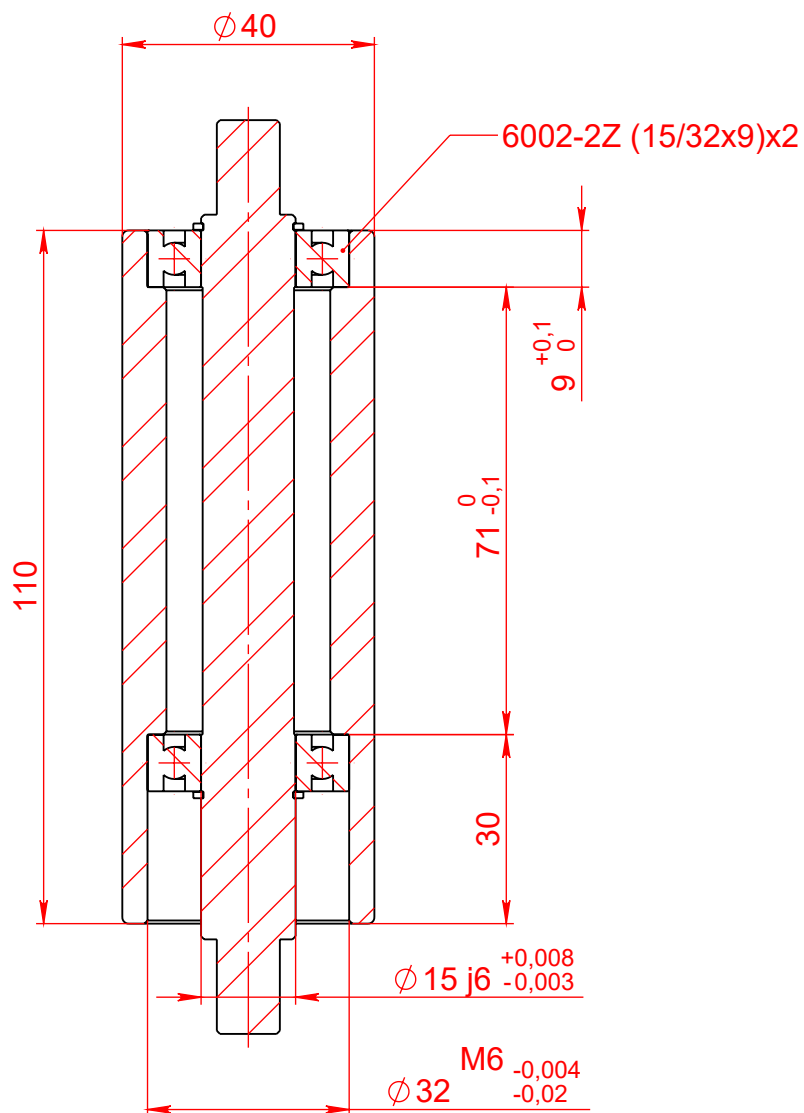
SECTION A-A SCALE 1 : 1.2
